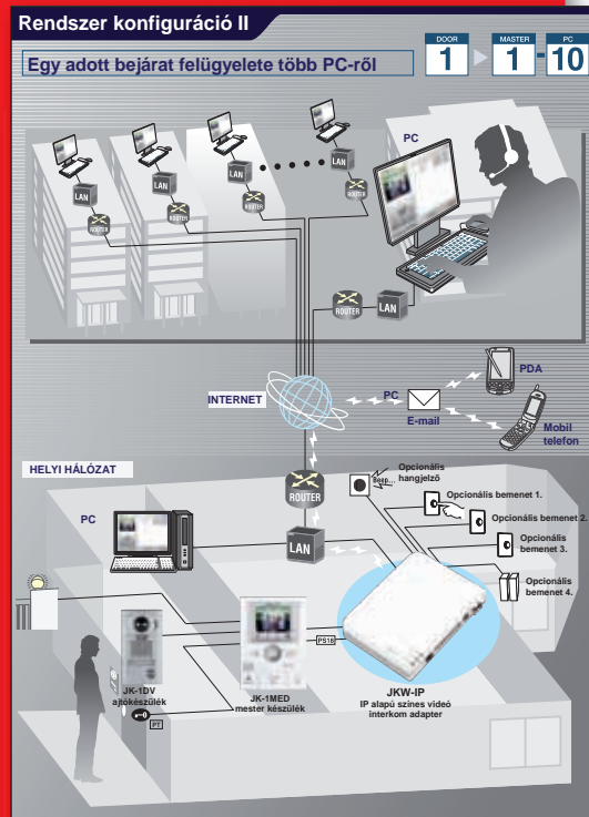
Az Aiphone JK/JKW-IP kaputelefon-rendszer konfigurációinak folyamatábrái
