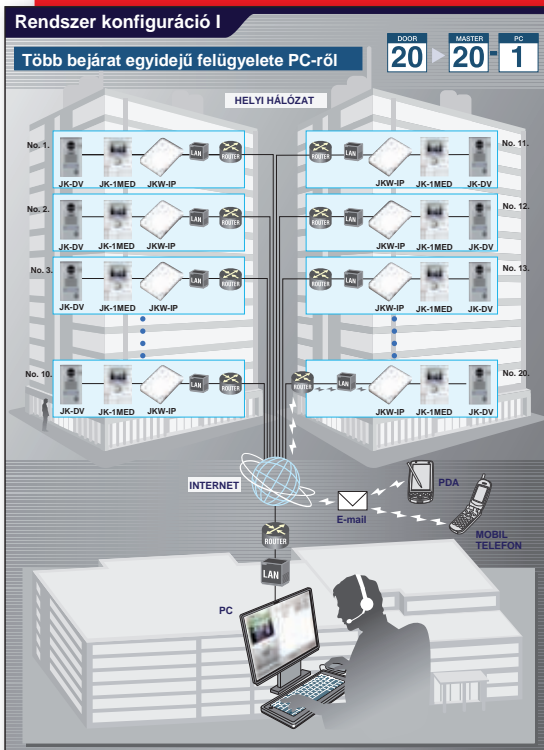
Az Aiphone JK/JKW-IP kaputelefon-rendszer konfigurációinak folyamatábrái
